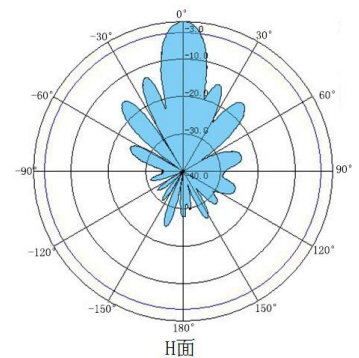
方向图
