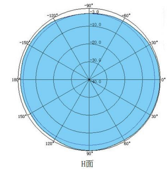
方向图
