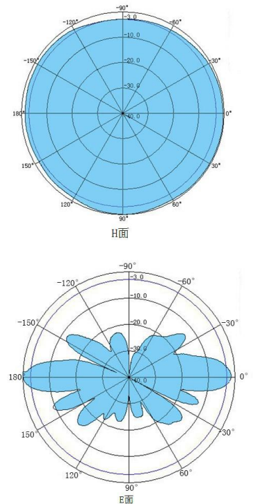
方向图
