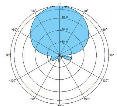
H面
