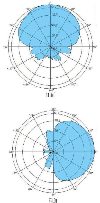
方向图
