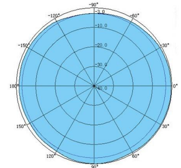
H面
