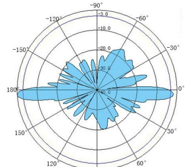
E面
