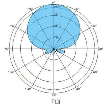
方向图
