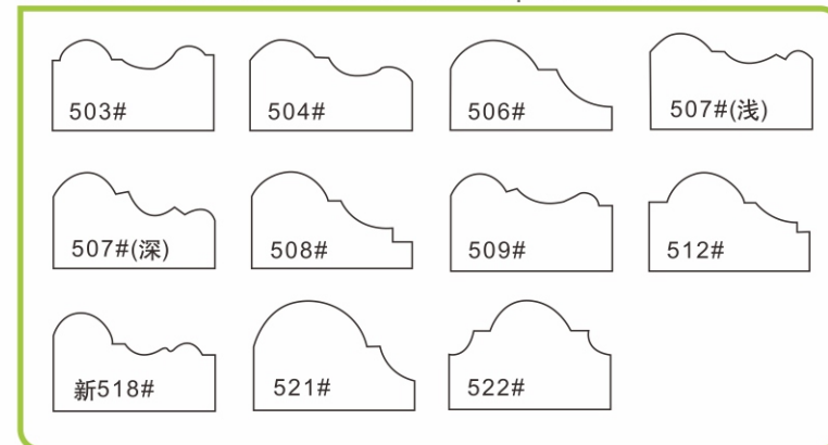
5公分系列电镀轮 5cm series electroplated wheels
