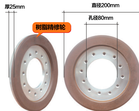
产品品牌: 博威工具 产品名称: 树脂结合轮 产品规格: 直径200mmx孔径80mmx厚25mm 使用范围: 瓷砖、陶瓷、玻化砖、微晶石、大理石、岩板砖
