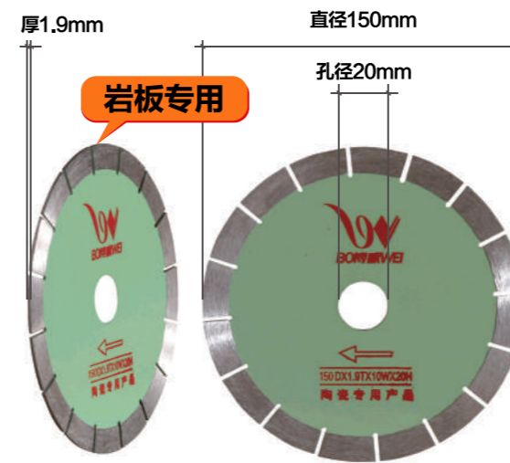
产品品牌：博威工具 产品名称：金刚石切割片 产品规格：直径150mmx孔径20mmx厚1.9mm 使用范围：瓷砖、陶瓷、玻化砖、微晶石、大理石、岩板砖
