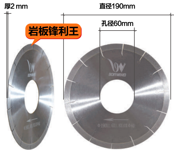
产品品牌: 博威工具 产品名称: 金刚石切割片 产品规格: 直径190mmx孔径60mmx厚1.9mm 使用范围: 瓷砖、陶瓷、玻化砖、微晶石、大理石、岩板砖
