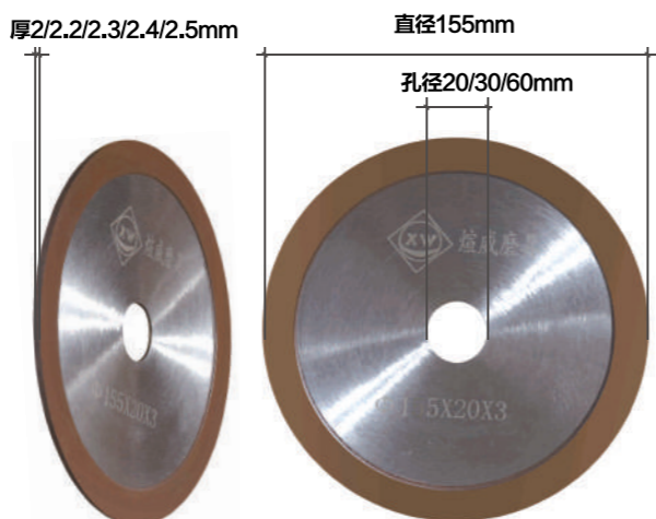
产品品牌: 煊威磨具 产品名称: 树脂结合开槽轮 产品规格: 直径155mmx孔径20/30/60mmx厚2.2/2.3/2.4/2.5mm 使用范围: 瓷砖、陶瓷、玻化砖、微晶石、大理石、岩板砖
