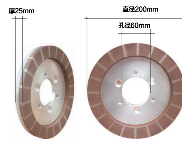
产品品牌: 博威工具 产品名称: 金刚树脂复合轮 产品规格: 直径200mmx孔径60x厚25mm 使用范围: 瓷砖、陶瓷、玻化砖、微晶石、大理石、岩板砖
