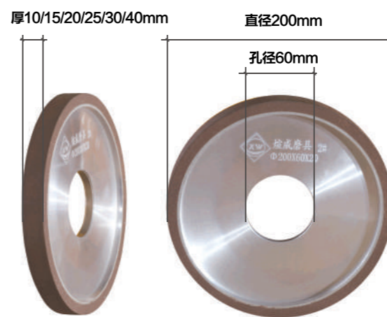
产品品牌: 煊威磨具 产品名称: 树脂结合轮 产品规格: 直径200mmx孔径60mmx厚10/15/20/25/30/40mm 使用范围: 瓷砖、陶瓷、玻化砖、微晶石、大理石、岩板砖
