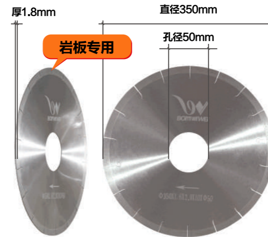
产品品牌: 博威工具 产品名称: 金刚石切割片 产品规格: 直径350mmx孔径50mmx厚1.8mm 使用范围: 瓷砖、陶瓷、玻化砖、微晶石、大理石、岩板砖
