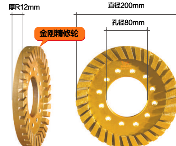
产品品牌: 博威工具 产品名称: 金刚石精修轮 产品规格: 直径200mmx孔径80mmx厚R25mm 使用范围: 瓷砖、陶瓷、玻化砖、微晶石、大理石、岩板砖
