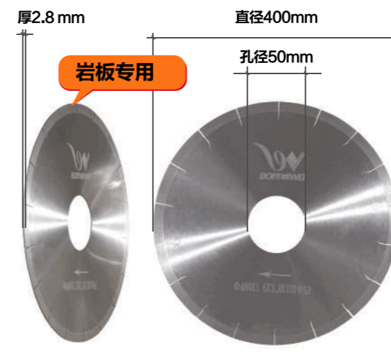
产品品牌: 博威工具 产品名称: 金刚石切割片 产品规格: 直径400mmx孔径50mmx厚2.8 mm 使用范围: 瓷砖、陶瓷、玻化砖、微晶石、大理石、岩板砖
