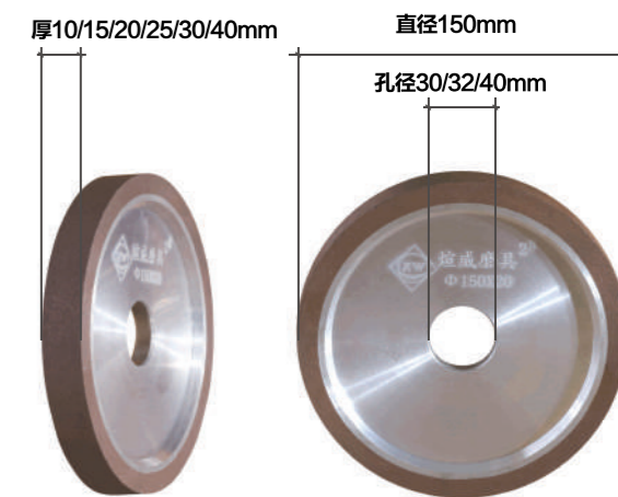
产品品牌: 煊威磨具 产品名称: 树脂结合轮 产品规格: 直径155mmx孔径30/32/40mmx厚10/15/20/25/30/40mm 使用范围: 瓷砖、陶瓷、玻化砖、微晶石、大理石、岩板砖
