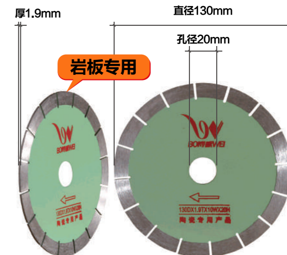
产品品牌：博威工具 产品名称：金刚石切割片 产品规格：直径130mmx孔径20mmx厚1.9mm 使用范围：瓷砖、陶瓷、玻化砖、微晶石、大理石、岩板砖
