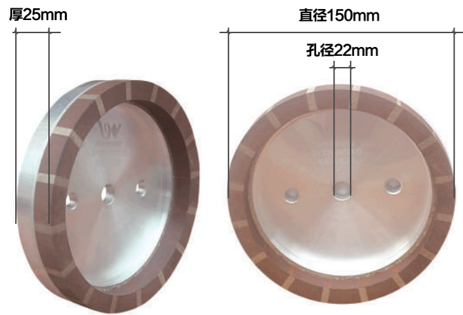
产品品牌：博威工具 产品名称：金刚树脂复合轮 产品规格：直径150mmx孔径22mmx厚25mm 使用范围：瓷砖、陶瓷、玻化砖、微晶石、大理石、岩板砖
