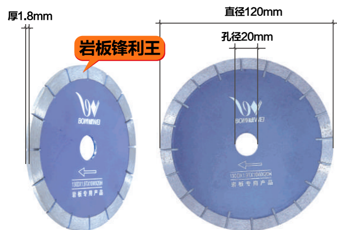
产品品牌：博威工具 产品名称：金刚石切割片 产品规格：直径120mmx孔径20mmx厚1.8mm 使用范围：岩板、陶瓷、玻化砖、微晶石、大理石、花岗岩 使用机型：云石机、角磨机
