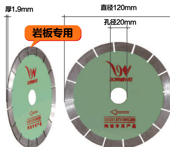
产品品牌：博威工具 产品名称：金刚石切割片 产品规格：直径120mmx孔径20mmx厚1.9mm 使用范围：瓷砖、陶瓷、玻化砖、微晶石、大理石、岩板砖
