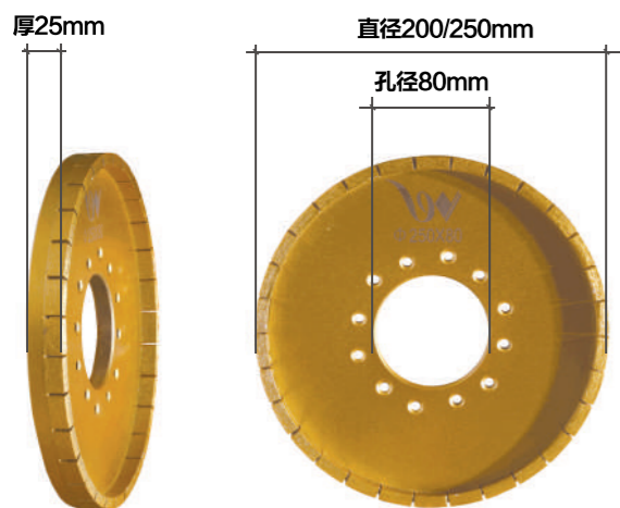
产品品牌: 博威工具 产品名称: 金刚石修边轮 产品规格: 直径200/250mmx孔径80mmx厚25mm 使用范围: 瓷砖、陶瓷、玻化砖、微晶石、大理石、岩板砖
