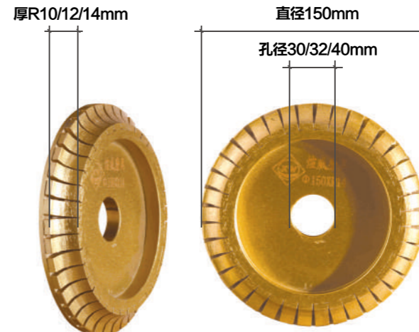
产品品牌: 博威工具 产品名称: 金刚石法国边磨轮 产品规格: 直径150mmx孔径30/32/40mmx厚R10/12/14mm 使用范围: 瓷砖、陶瓷、玻化砖、微晶石、大理石、岩板砖
