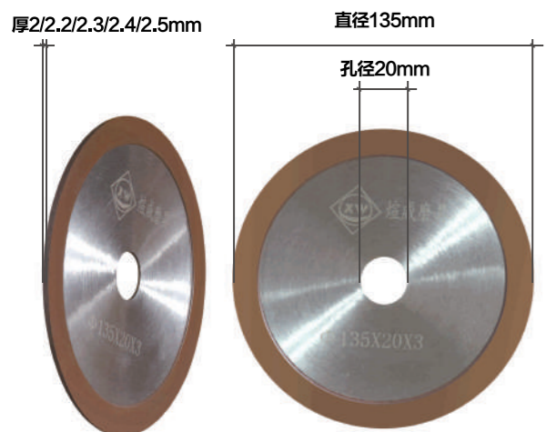
产品品牌: 煊威磨具 产品名称: 树脂结合开槽轮 产品规格: 直径150mmx孔径20mmx厚2.2/2.3/2.4/2.5mm 使用范围: 瓷砖、陶瓷、玻化砖、微晶石、大理石、岩板砖
