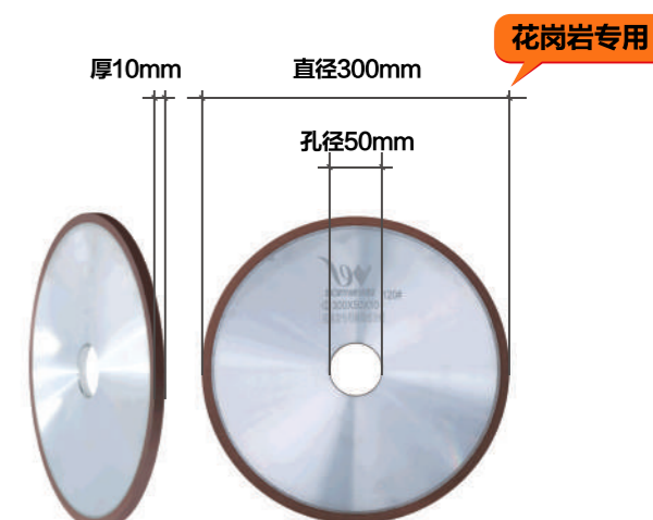
产品品牌: 博威工具 产品名称: 树脂开槽轮 产品规格: 直径300mmx孔径50mmx厚10mm 使用范围: 岩板、陶瓷、玻化砖、微晶石、大理石、花岗岩
