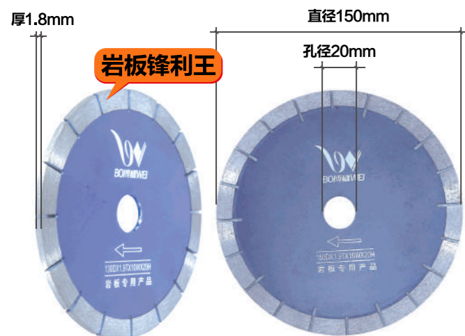
产品品牌：博威工具 产品名称：金刚石切割片 产品规格：直径150mmx孔径20mmx厚1.8mm 使用范围：岩板、陶瓷、玻化砖、微晶石、大理石、花岗岩 使用机型：云石机、角磨机
