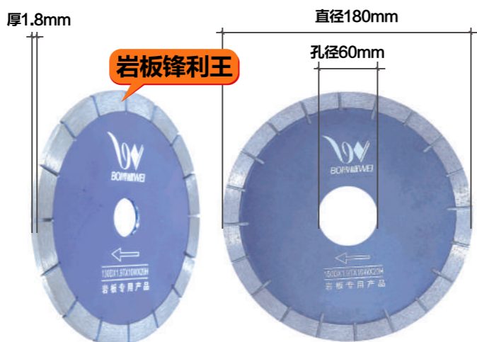
产品品牌：博威工具 产品名称：金刚石切割片 产品规格：直径180mmx孔径60mmx厚1.8mm 使用范围：岩板、陶瓷、玻化砖、微晶石、大理石、花岗岩 使用机型：云石机、角磨机
