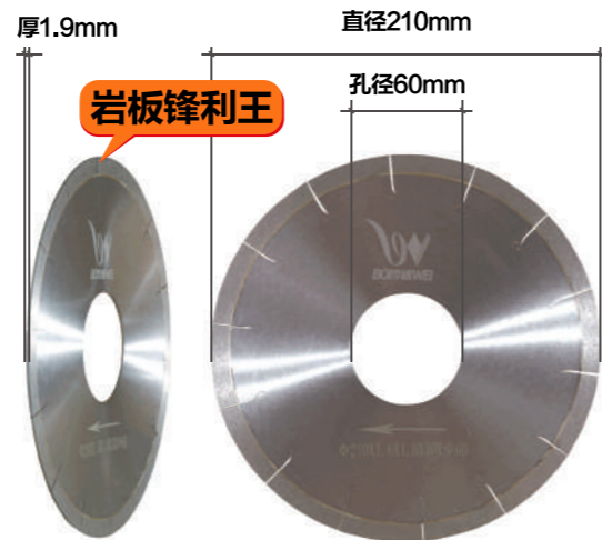
产品品牌: 博威工具 产品名称: 金刚石切割片 产品规格: 直径210mmx孔径60mmx厚1.9mm 使用范围: 瓷砖、陶瓷、玻化砖、微晶石、大理石、岩板砖
