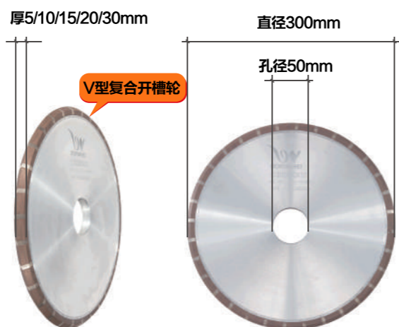
产品品牌: 博威工具 产品名称: V金刚树脂复合轮 产品规格: 直径300mmx孔径50mmx厚5/10/15/20/30mm 使用范围: 岩板、陶瓷、玻化砖、微晶石、大理石、花岗岩
