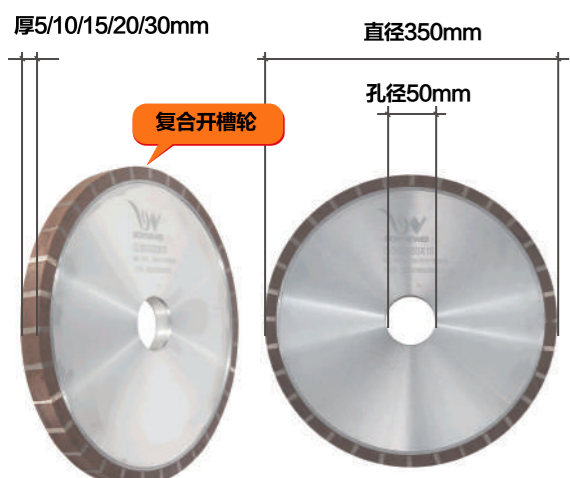
产品品牌: 博威工具 产品名称: 金刚树脂复合轮 产品规格: 直径350mmx孔径50mmx厚5/10/15/20/30mm 使用范围: 岩板、陶瓷、玻化砖、微晶石、大理石、花岗岩
