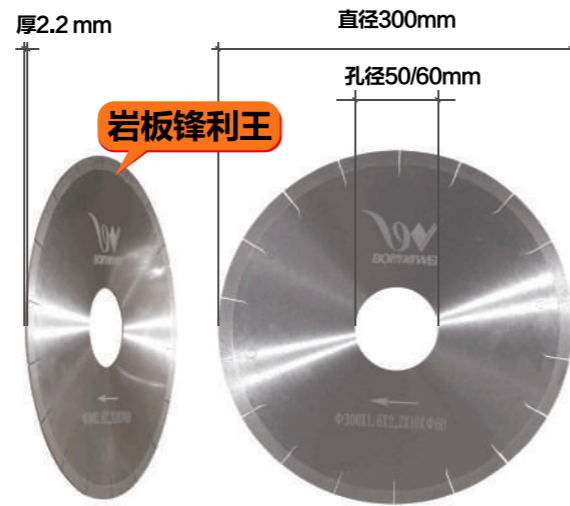
产品品牌: 博威工具 产品名称: 金刚石切割片 产品规格: 直径300mmx孔径50/60mmx厚2.2 mm 使用范围: 瓷砖、陶瓷、玻化砖、微晶石、大理石、岩板砖
