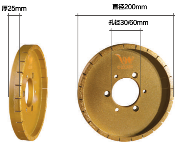
产品品牌: 博威工具 产品名称: 金刚石修边轮 产品规格: 直径200mmx孔径30/60mmx厚25mm 使用范围: 瓷砖、陶瓷、玻化砖、微晶石、大理石、岩板砖
