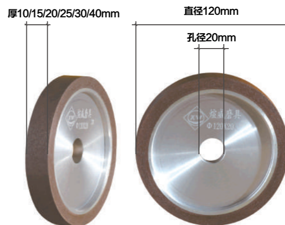
产品品牌: 煊威磨具 产品名称: 树脂结合轮 产品规格: 直径120mmx孔径20mmx厚10/15/20/25/30/40mm 使用范围: 瓷砖、陶瓷、玻化砖、微晶石、大理石、岩板砖
