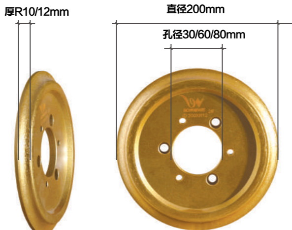
产品品牌: 博威工具 产品名称: 陶瓷圆角轮 产品规格: 直径200mmx孔径30/60/80mmx厚R10/12mm 使用范围: 瓷砖、陶瓷、玻化砖、微晶石、大理石、岩板砖
