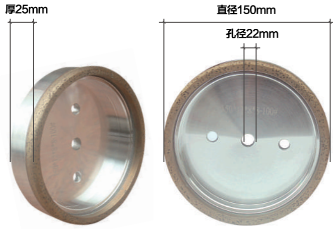
产品品牌：博威工具 产品名称：青铜结合玻璃轮 产品规格：直径150mmx孔径22mmx厚25mm 使用范围：瓷砖、陶瓷、玻化砖、微晶石、大理石、岩板砖
