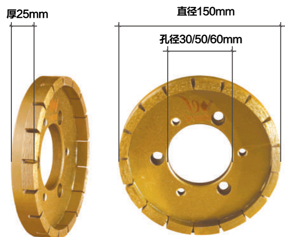
产品品牌: 博威工具 产品名称: 金刚石修边轮 产品规格: 直径150mmx孔径30/50/60x厚25mm 使用范围: 瓷砖、陶瓷、玻化砖、微晶石、大理石、岩板砖
