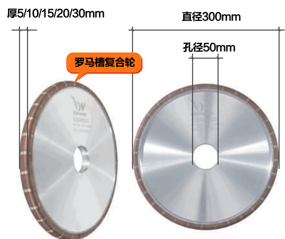
产品品牌: 博威工具 产品名称: 金刚树脂复合轮 产品规格: 直径300mmx孔径50mmx厚5/10/15/20/30mm 使用范围: 岩板、陶瓷、玻化砖、微晶石、大理石、花岗岩
