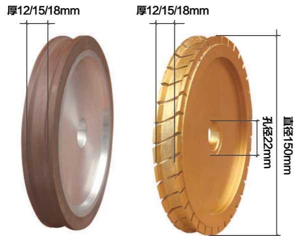
产品品牌：博威工具 产品名称：岩板倒角轮 产品规格：直径150mmx孔径22mmx厚12/15/18mm 使用范围：瓷砖、陶瓷、玻化砖、微晶石、大理石、岩板砖
