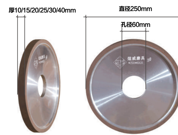
产品品牌: 煊威磨具 产品名称: 树脂结合轮 产品规格: 直径250mmx孔径60mmx厚10/15/20/25/30/40mm 使用范围: 瓷砖、陶瓷、玻化砖、微晶石、大理石、岩板砖
