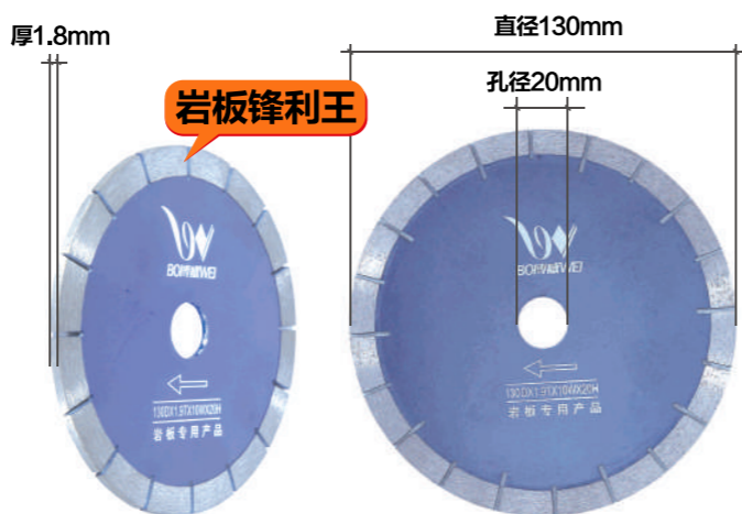
产品品牌：博威工具 产品名称：金刚石切割片 产品规格：直径130mmx孔径20mmx厚1.8mm 使用范围：岩板、陶瓷、玻化砖、微晶石、大理石、花岗岩 使用机型：云石机、角磨机
