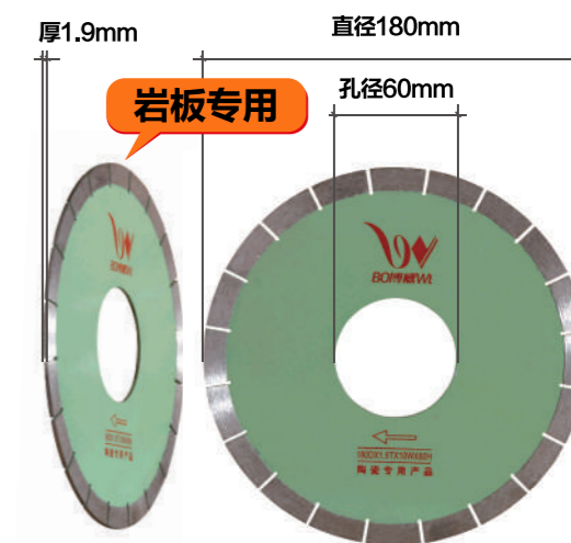
产品品牌：博威工具 产品名称：金刚石切割片 产品规格：直径180mmx孔径60mmx厚1.9mm 使用范围：瓷砖、陶瓷、玻化砖、微晶石、大理石、岩板砖
