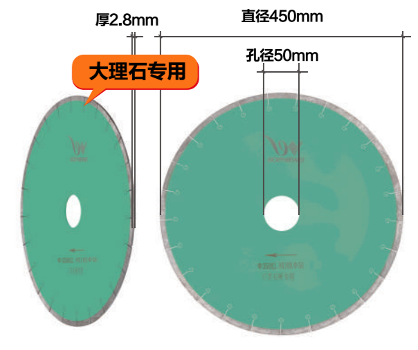
产品品牌: 博威工具 产品名称: 金刚石切割片 产品规格: 直径450mmx孔径50mmx厚2.8mm 使用范围: 瓷砖、陶瓷、玻化砖、微晶石、大理石、岩板砖
