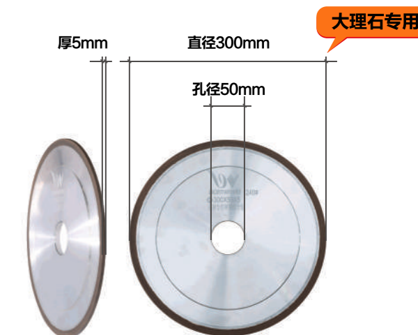
产品品牌: 博威工具 产品名称: 树脂开槽轮 产品规格: 直径300mmx孔径50mmx厚5mm 使用范围: 岩板、陶瓷、玻化砖、微晶石、大理石、花岗岩
