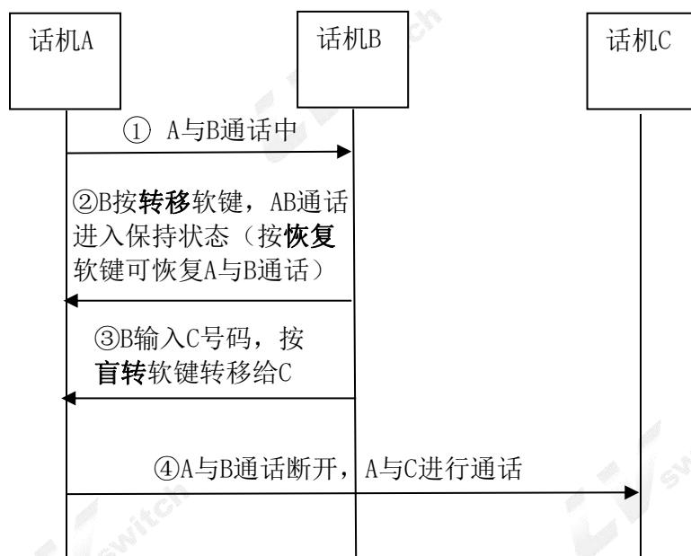
盲转流程图
