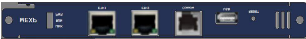
图 1-4 IP PBX6000 MEXP 主机扩展管理板外观图
