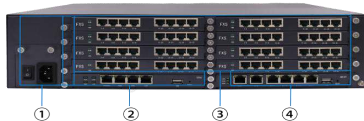
图 1-1 IP PBX6000 前面板图
