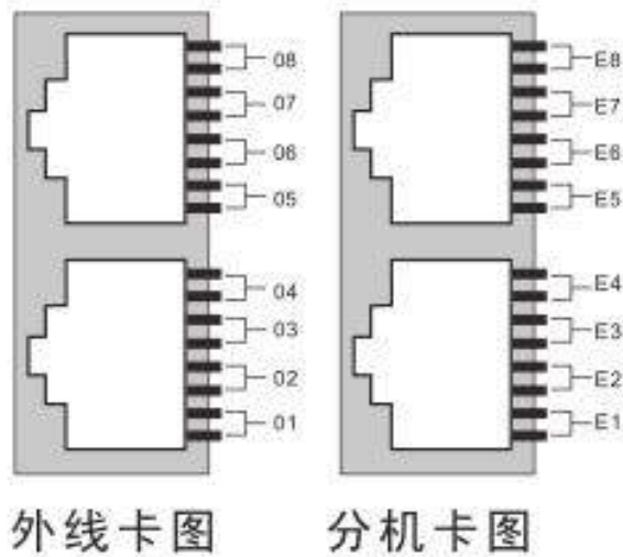
RJ45 接口顺序概览图
