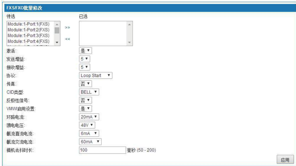
图 6-128 模拟接口配置-FXS/FXO 批量修改
